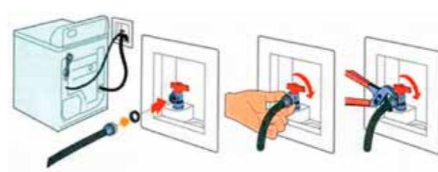
Присоединить заливную трубку к запорному крану
