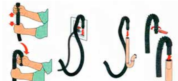
Присоединить сливную трубу к канализации (при необходимости подрезать конусный наконечник)
