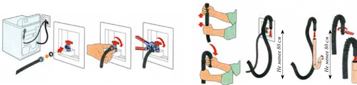
Присоединить заливную трубку к запорному крану
